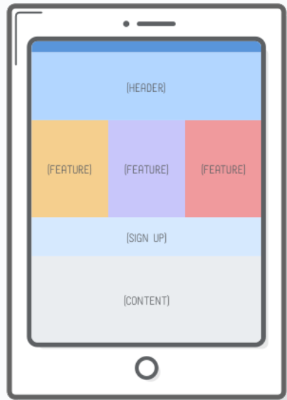
ZOOM ENABLED
